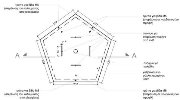
κάτοψη γαλβανισμένου φύλλου 3mm
