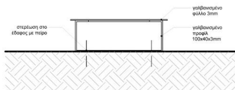
τομή AA
