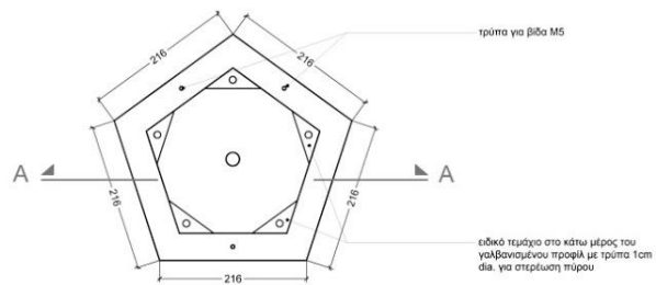
κάτοψη γαλβανισμένου προφίλ 100x40x3mm
