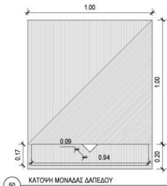
50 ΚΑΤΩΝΗ ΜΟΝΑΔΑΣ ΔΑΠΕΔΟΥ ΚΛΙΜΑΚΑ 1:20
