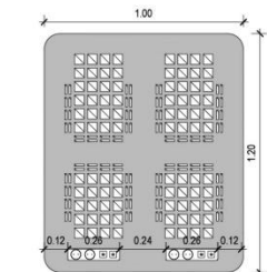
40 ΚΑΤΩΝΗ ΠΑΝΕΛΣ ΜΕ ΤΡΥΠΕΣ ΓΙΑ ΗΛ. ΠΑΡΟΧΕΣ ΚΛΙΜΑΚΑ 1:20
