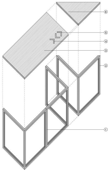
10 ΑΞΟΝΟΜΕΤΡΙΚΟ ΣΧΕΔΙΟ ΑΤΟΜΙΚΟΥ ΓΡΑΦΕΙΟΥ ΚΛΙΜΑΚΑ 1:20
