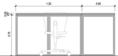
50 ΕΜΠΡΟΣΘΙΑ ΟΝΗ ΑΤΟΜΙΚΟΥ ΓΡΑΦΕΙΟΥ ΚΛΙΜΑΚΑ 1:20
