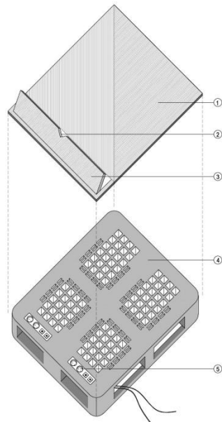
10 ΑΞΟΝΟΜΕΤΡΙΚΟ ΣΧΕΔΙΟ ΜΟΝΑΔΑΣ ΔΑΠΕΔΟΥ ΚΛΙΜΑΚΑ 1:20
